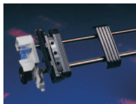
Traktorový podavač
